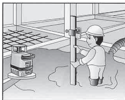
生コン打設
